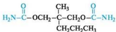
мепротан (мепробамат)
