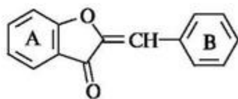
ауроны
