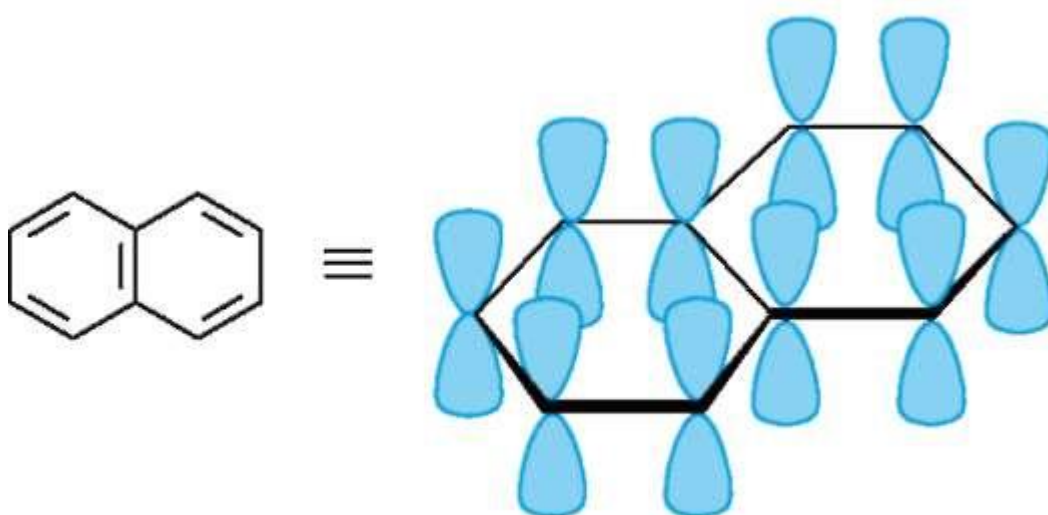
нафталин, 10 \pi -электронов ( n = 2 )
