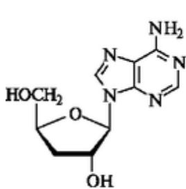
кордицепин
