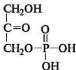
дигидроксиацетонфосфат
