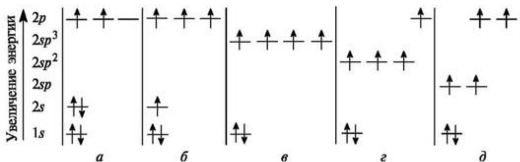
Рис. 2.1. Распределение электронов по орбиталям у атома углерода в основном (а), возбужденном (б) и гибридных состояниях (в - sp^3 , г - sp^2 , д - sp )
