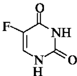
5-фторурацил
