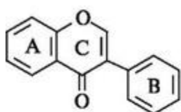
изофлавоны
