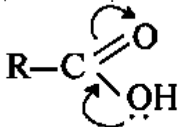
карбоновая кислота
