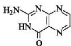
2-аминоптеридин-4-он (фрагмент фолиевой кислоты)
