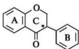
изофлаваноны
