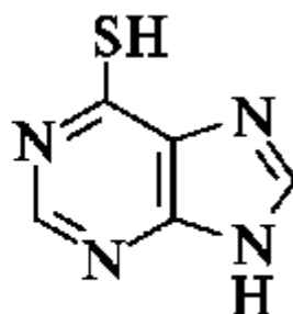
6-меркаптопурин
