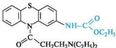
этацизин
