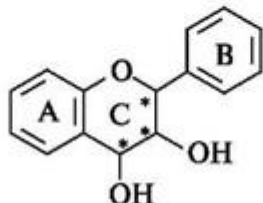
флаван-3,4-диолы
