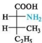
D-изолейцин
