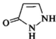
пиразолон
