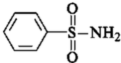
бензолсульфонамид
